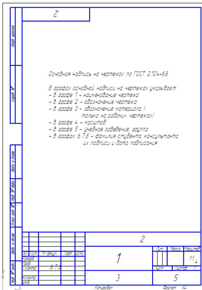
Рисунок 4 Основная надпись на чертежах (форма 1 ГОСТ 2.104-68)
